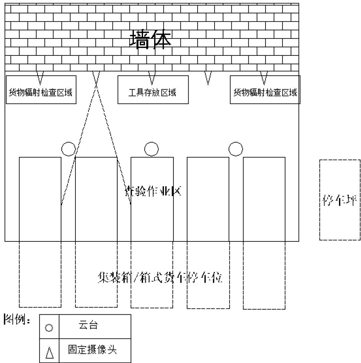
图 A.1 单侧查平台/场地设置（平面图）
