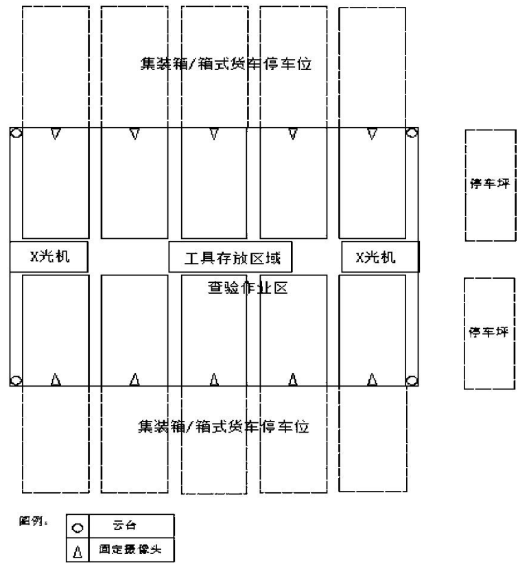
图 A.3 双侧查验平台/场地设置（平面图）
