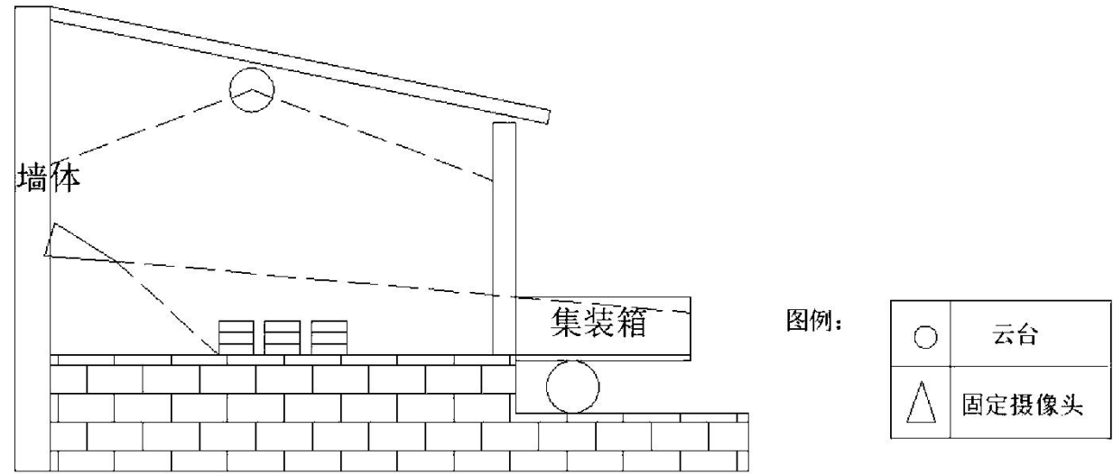
图 A.2 单侧查验平台/场地设置（立面图）
